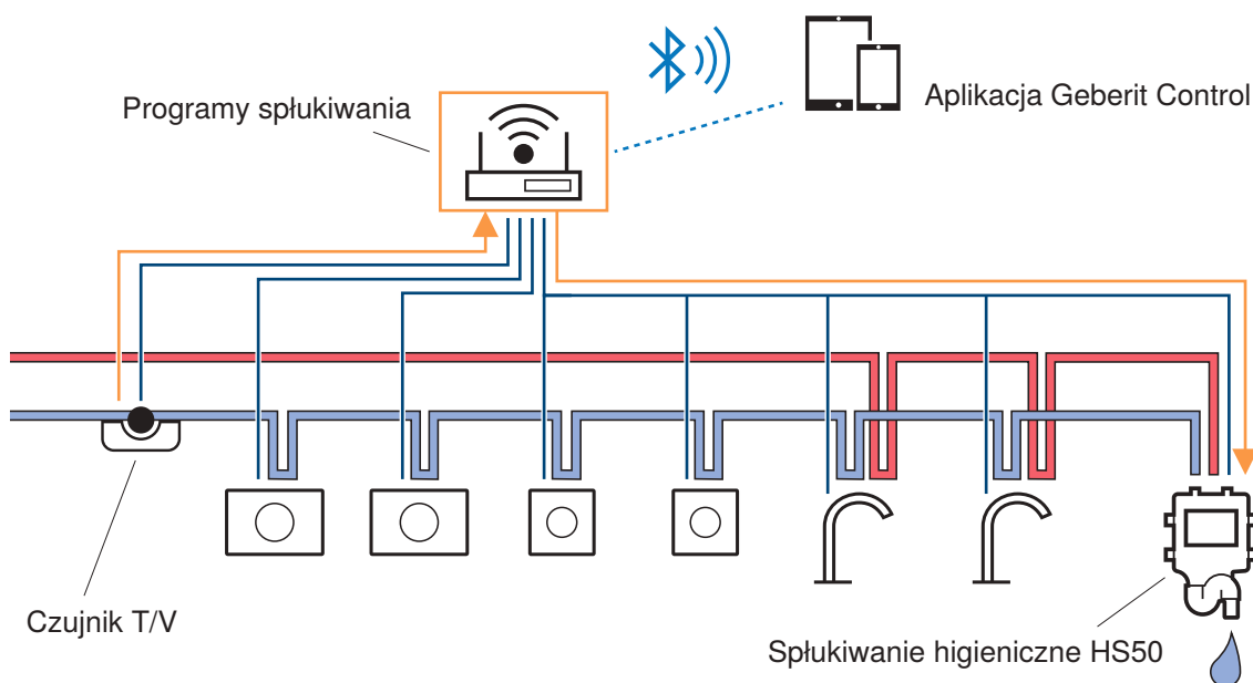
Rysunek 20: Przykład: Geberit Gateway z programami spłukiwania w trybie pracy sieciowej. Czujnik przepływu (czujnik T/V) rejestruje ilość wody spłukującej w programach spłukiwania w Gateway. Programy spłukiwania sterują spłukiwaniem higienicznym HS50.
