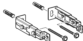
111.064.00.1 Zestaw do mocowania nóg stelaża do ściany
