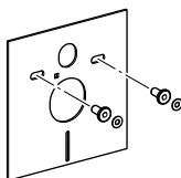
156.050.00.1 Zestaw do izolacji akustycznej do wiszącej misk i bidetu Geberit
